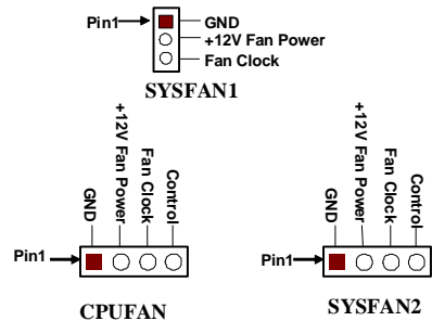
FAN Headers
