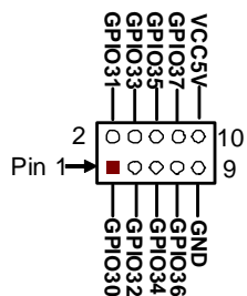
GPIO_CON Header
