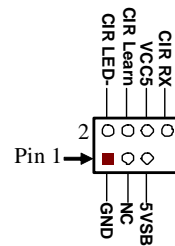
CIR Header
