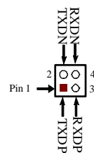
TX-RXCOM6 Header
