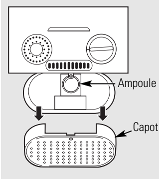
Emplacement de la lampe dans un réfrigérateur de 10 pi 3
