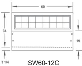
SW60-12C
