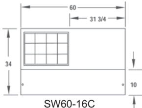
SW60-16C
