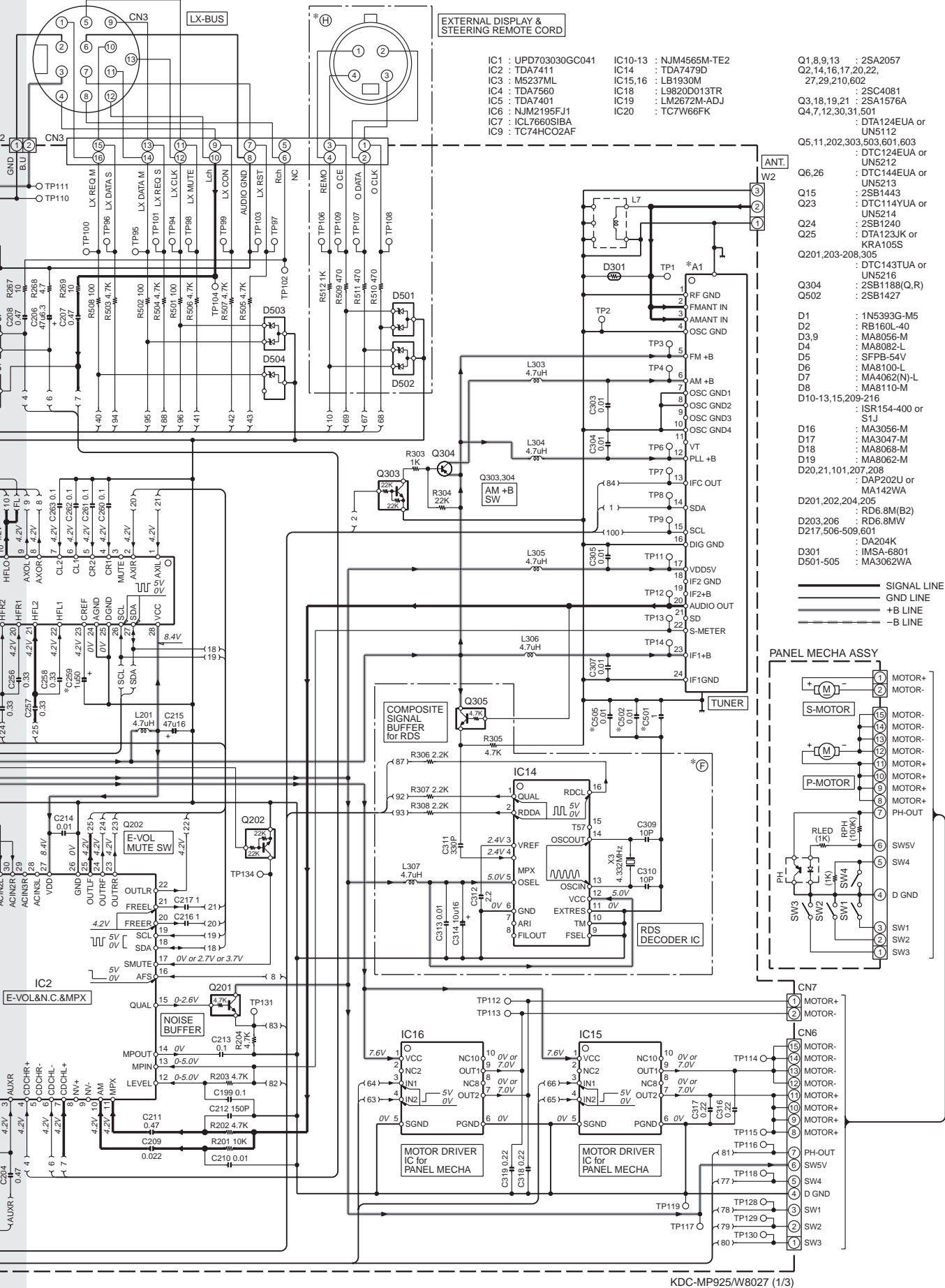
KDC-MP925/W8027 (1/3)
