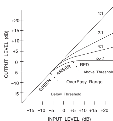
Figura 2: Curva de compresión OverEasy y los LED de umbral
