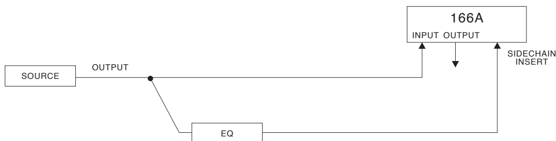
Abb. 3: Frequenzselektive Kompression
