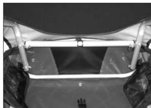
Ansicht fertig montierte Teleskopstange von innen
