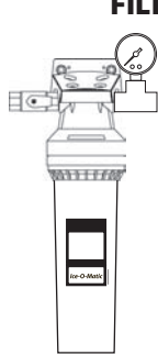
IFQ1 15"H x 6"W x 4"D (381 x 152 x 102 mm)
