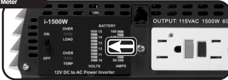
Volts Meter
