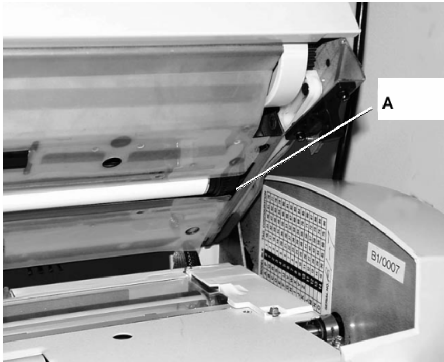
A: Calibration Roll Drive Gear
