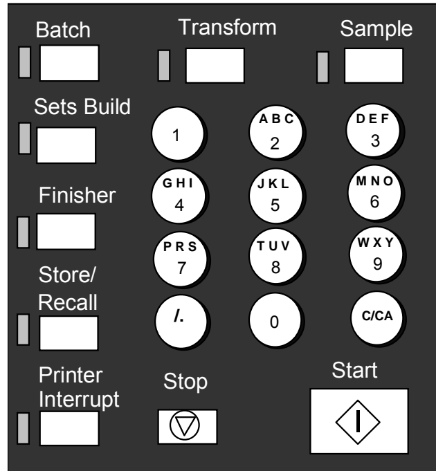
Numeric Keypad
