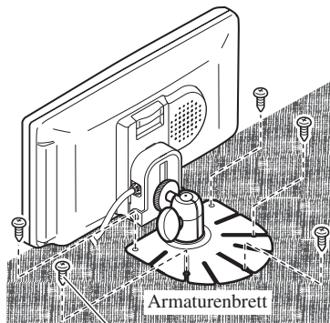
Schneidschrauben (3 × 12 mm)
