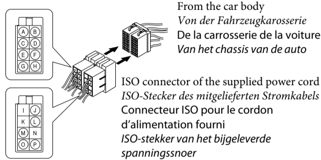
View from the lead side Von der Kabelseite aus gesehen Vue à partir du côté des fils Gezien vanaf de spanningstoevoerkant
