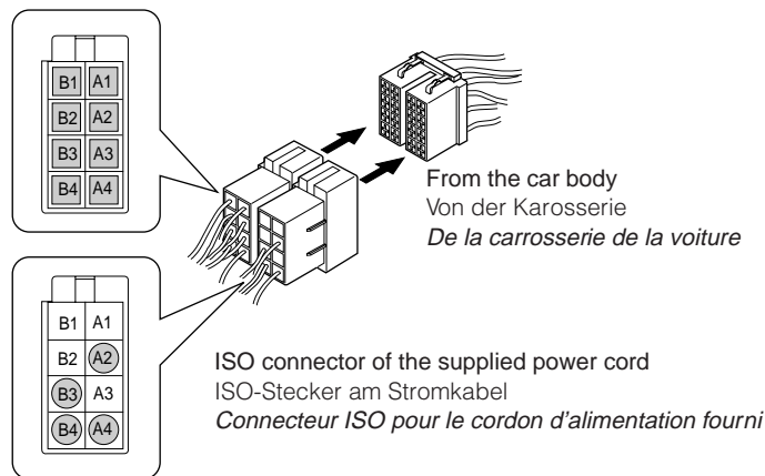
View from the lead side Ansicht von der Leitungsseite Vue à partir du côté des fils
