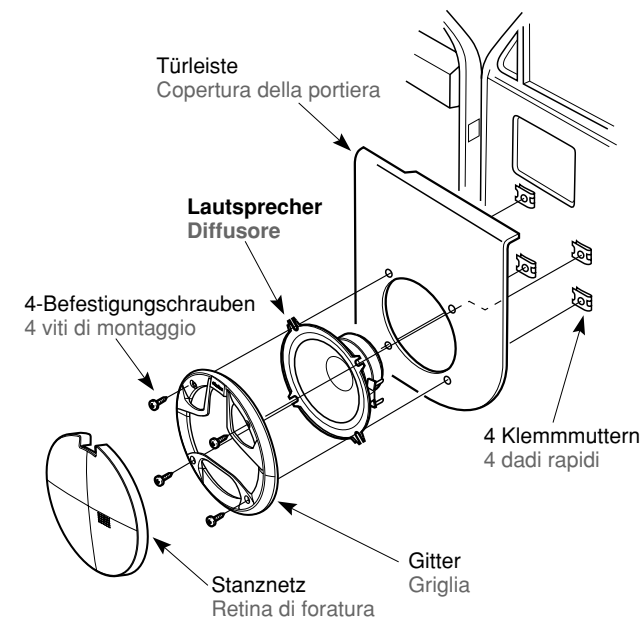
Abbildung 4 / Figura 4 (SRQ1320S)
