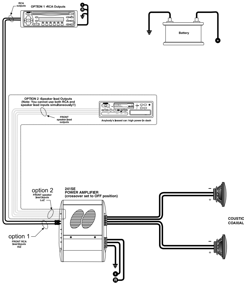
Figure 6 : Installation traditionnelle
