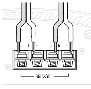
Figure 9 : mode stéréo.
