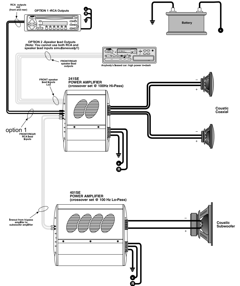
Figure 7 : Système multi amplifié
