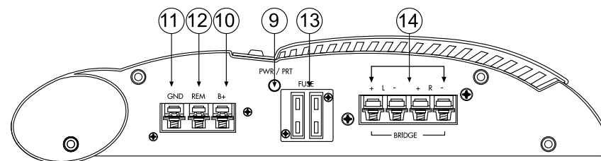
Figure 2: Panneau des sorties et des indicateurs
