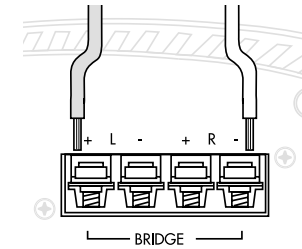
Figure 10 : mode ponté sur un seul subwoofer de 4 ohms
