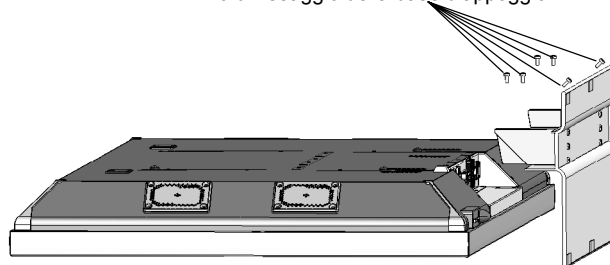
Viti di fissaggio della base d'appoggio
