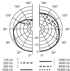
Diagrama polar
