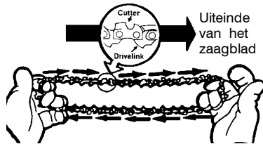
JUISTE KETTINGRICHTING
