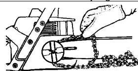
Plaats de ketting op het tandwiel
