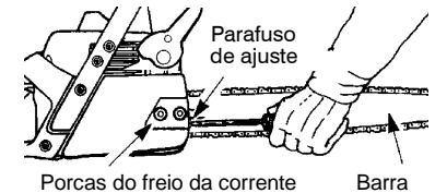
Parafuso de ajuste - 1/4 de volta
