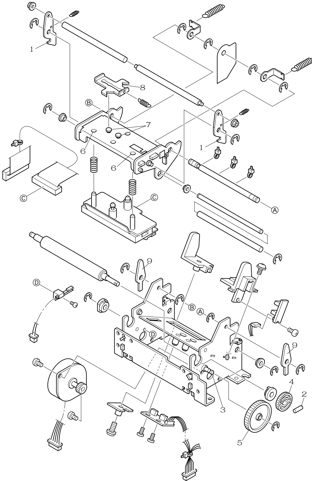
Fig. 4-1 Lubrication Points
