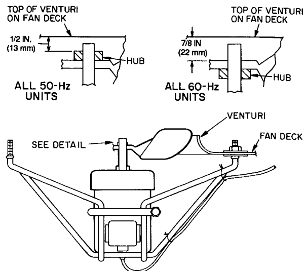
Fig. 31 — Condenser Fan Adjustment
