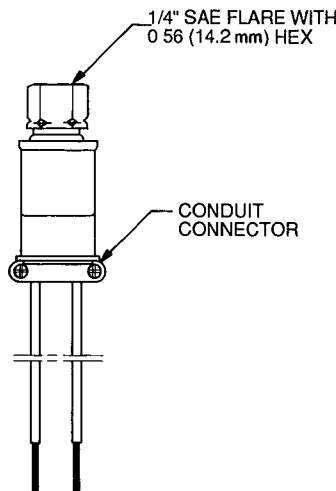
Fig. 15 — Fan Cycle Pressure Switch
