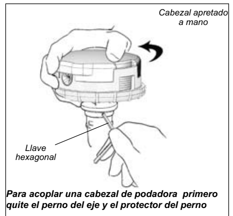
Inserte el lado más largo de la llave hexagonal a través de ambas muescas
