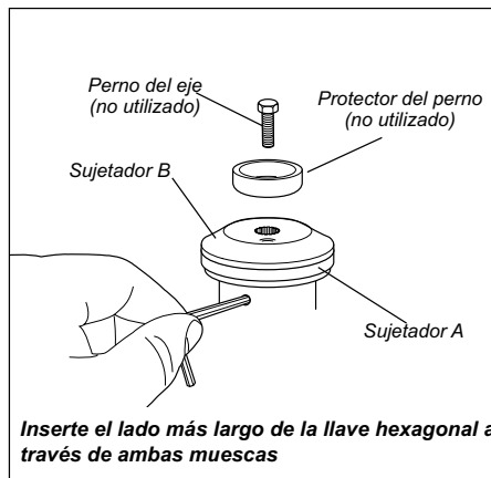
Para acoplar una cabezal de podadora primero quite el perno del eje y el protector del perno
