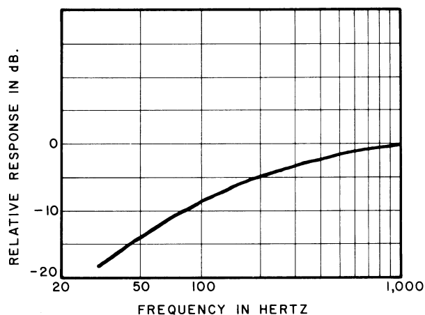
HOCHPASSFILTER-AKTION ABBILDUNG 1
