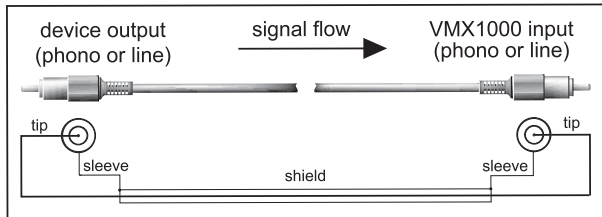
Fig. 3.5: RCA cable
