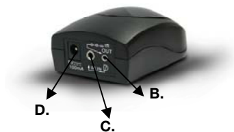
B. IR probes output connection
