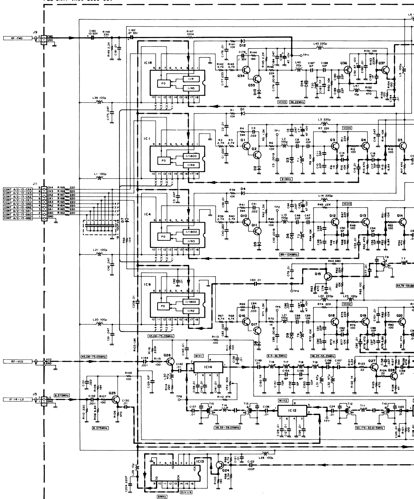
PLL UNIT (X50-2050-00)
