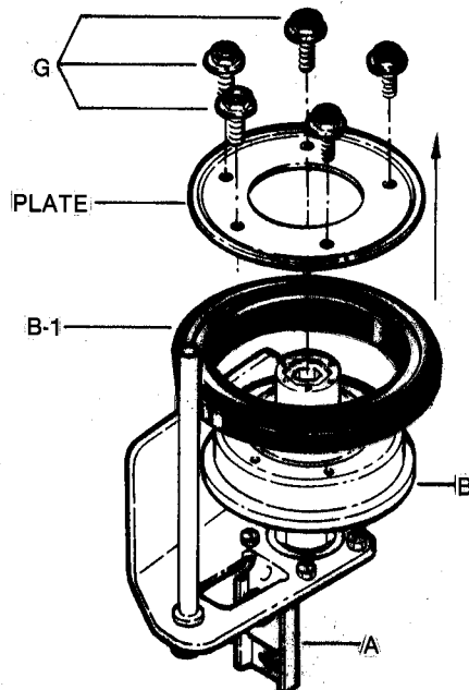
FIG. 15 -DRIVEN DISC
