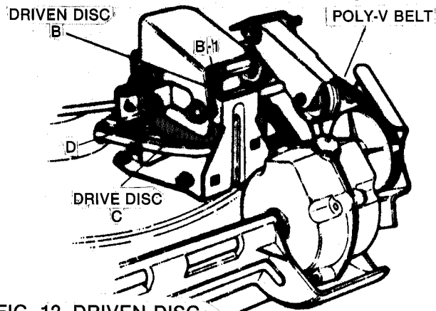
FIG. 12 -DRIVEN DISC
