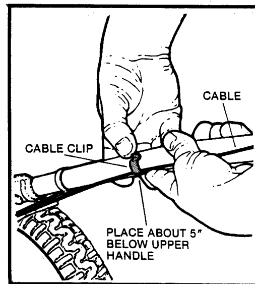
FIG. 11-A - CABLE CLIP
