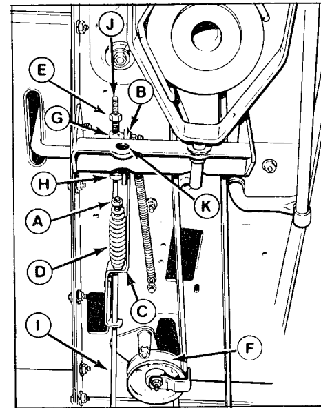
A. Nut B. Slot (in brake rod guide) C. Brake Rod Guide D. Spring E. Nut F. Idler Pulley G. Clutch Rod Guide H. Set Collar I. Brake Rod J. Clutch Rod K. Hole, 3/4" Dia.
