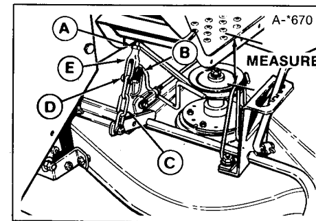
A. Nut B. Clip C. Chain D. PIN E. Clevis
