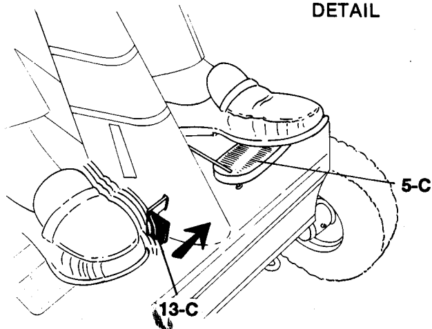
FIG. 1-A CLUTCH/BRAKE DETAIL
