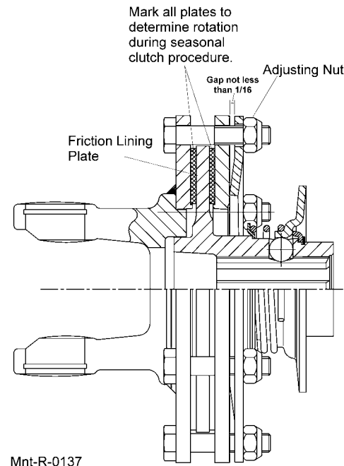
Disc Spring Clutch (2) (Belleville)
