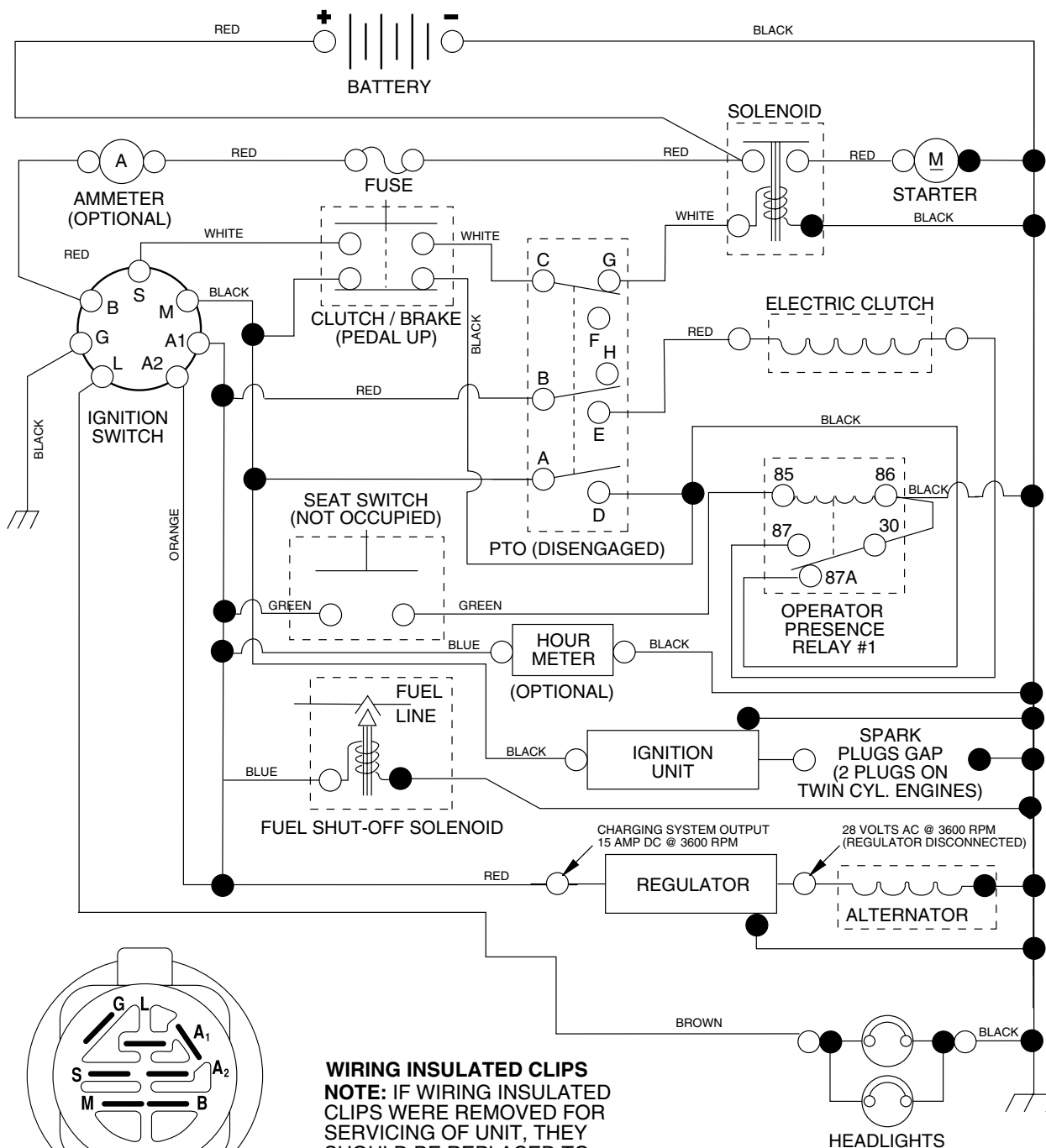
PTO SWITCH
