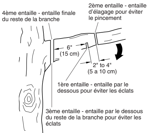
Figure 18 - Coupe d'une branche
