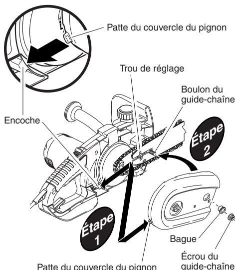
Figure 7 - Installation du couvercle du pignon
