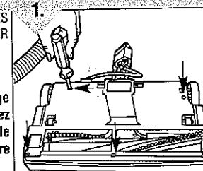
Schéma 1 Enlevez le dispositif de protection du suceur. Les flèches indiquent l'emplacement des vis.
