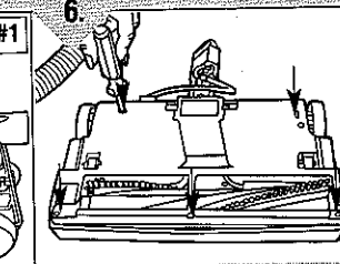
Schéma 6 Remettez en place le dispositif de protection du suceur. Retournez le suceur motorisé et remettez les cinq (5) vis.
