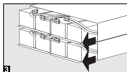
3 Retirer les batteries internes (Glisser hors du boîtier du bloc-batterie)
