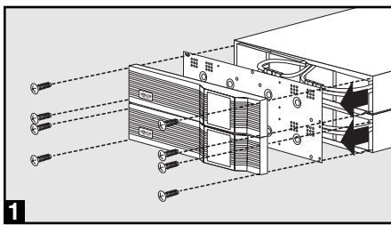
1 Desatornilla y Remueva el Panel Frontal del Módulo de Baterías y la Tapa de la Batería
