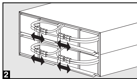
2 Desconecte las Baterías Internas (4 Pares de Conectores Rojo/Negro)
