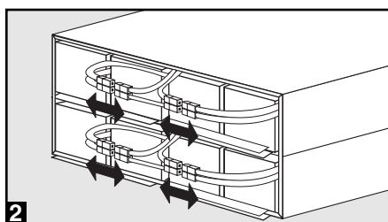
2 Déconnecter les batteries internes (4 ensembles de connecteurs rouge/noir)
