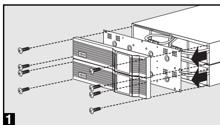
1 Dévisser et retirer le panneau avant du bloc-batterie et la plaque de protection des batteries
