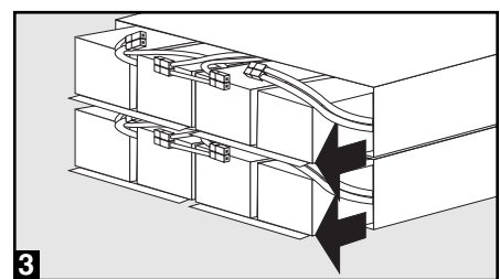
3 Remueva las Baterías Internas (Deslícelas del Gabinete del Módulo de Baterías)
