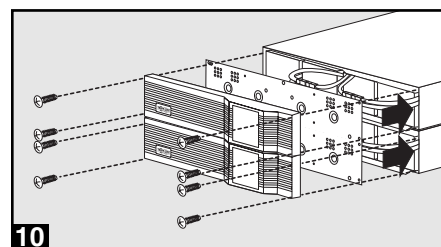
10 Reposer la plaque de protection des batteries et le panneau avant du bloc-batterie (Visser en place)
