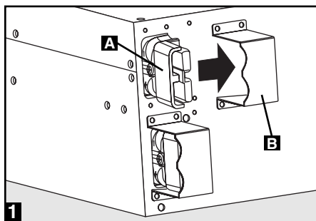
1 Retirer les ferrures de retenue B d'un des connecteurs du bloc-batterie externe du module d'alimentation de l'onduleur et d'un des connecteurs du panneau arrière du bloc-batterie A .
