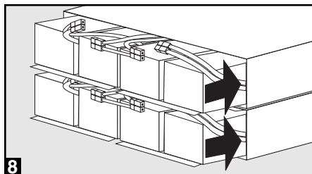
8 Insérer les batteries internes (glisser dans le boîtier du bloc-batterie)
