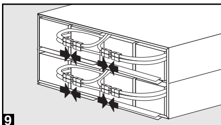
9 Connecter les 4 ensembles de connecteurs rouge/noir des batteries internes (connecter noir au noir et rouge au rouge.)
