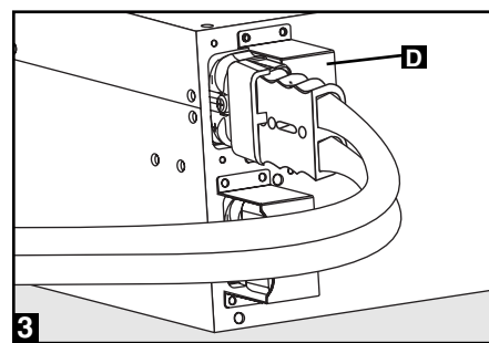
3 Fixer les ferrures de retenue D à droite de chaque connecteur, à l'aide des trous existants à la droite de l'emplacement original de la ferrure.
