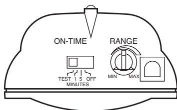
Parte inferior del detector
