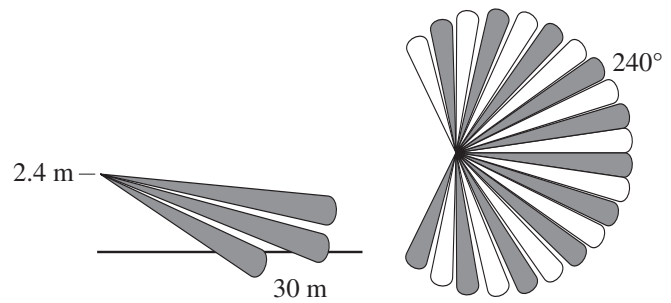
Figura 2: Ángulos de Protección
