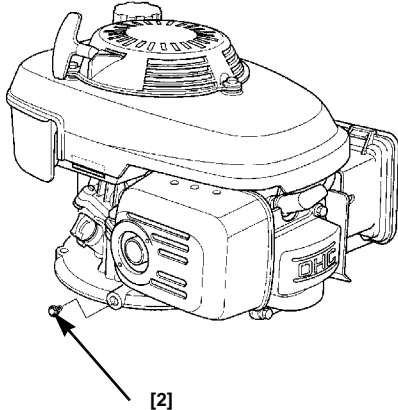
AVEC VIS DE DÉCHARGE
