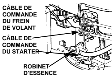
TYPE 4 : STARTER À RETOUR AUTOMATIQUE/CARBURATEUR PRÉRÉGLÉ
