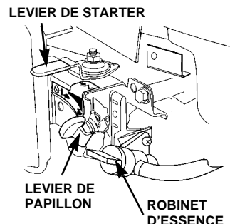
TYPE 3 : FREIN DE VOLANT/STARTER COMMANDÉ/CARBURATEUR PRÉRÉGLÉ
