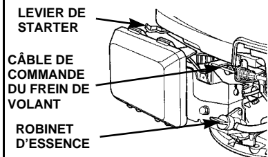
TYPE 4 : STARTER À RETOUR AUTOMATIQUE/CARBURATEUR PRÉRÉGLÉ
