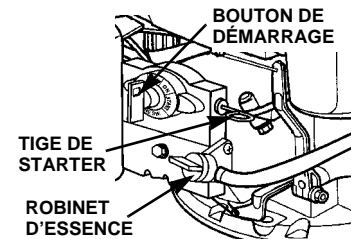
TYPE 7 : DÉMARREUR ÉLECTRIQUE (À BOUTON DE DÉMARRAGE)/STARTER MANUEL/CARBURATEUR PRÉRÉGLÉ
