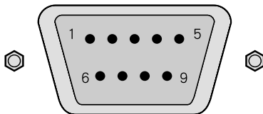
RS-232C terminal (RS-232C)
