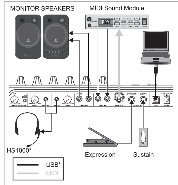
Fig. 1.3: Hookup example
